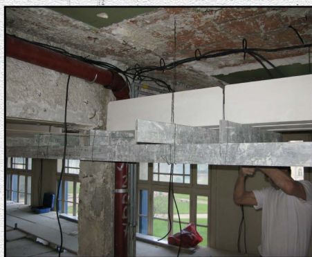
Mise en place des nouvelles poutres moulées - Janvier 2008 -
